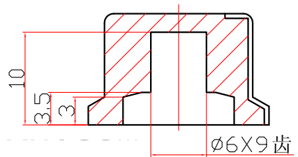
SEC.A-A
