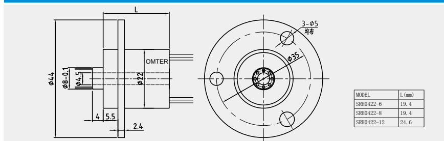
外形尺寸 OUTLINE DIMENSION 单位 (UNIT) mm
